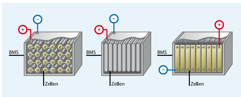
Aufbau von Zellmodulen aus zylindrischen (links), Pouch- (mitte) und prismatischen Zellen
