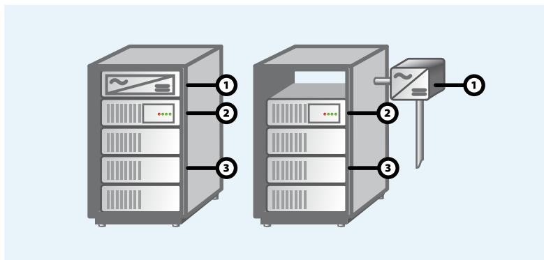
Prinzipielle Typen von Solarstrom-Speichersystemen (links: mit integriertem Wechselrichter; rechts: mit externem Wechselrichter)
