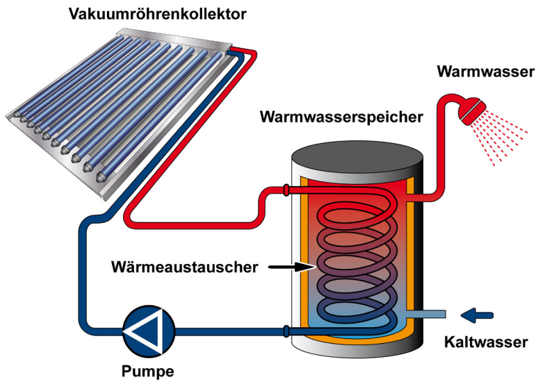
Abb. 4 Aufbau Solaranlage
