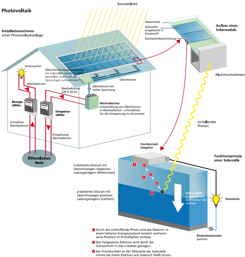
Abb. 12 Funktionsweise einer PV-Anlage
